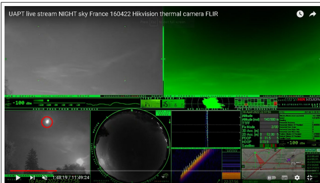
5) Possible fireball
