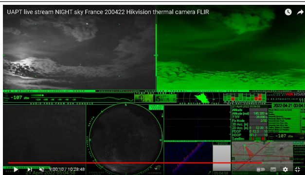
4) Meteor flash
